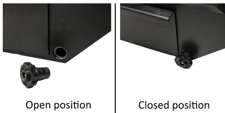
Kuva 5. Ulkokamiinan tyhjennystulppa
